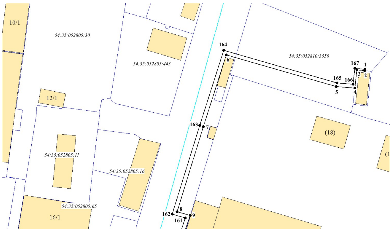
Выносной лист 1
